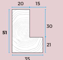
L FRAME 4007A
