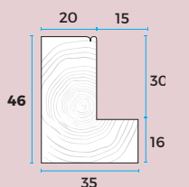
L FRAME 4001A
