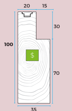
100mm L FRAME F/F 4008T
