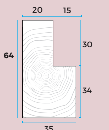
64mm L FRAME 4007B
