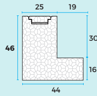
46mm L FRAME F/F P4008K
