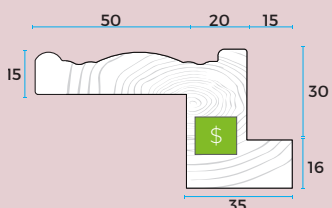
DECO Z FRAME 4004
