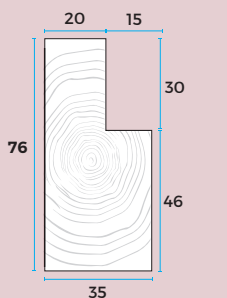
76mm L FRAME 4007C
