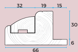
DECO L FRAME F/F 4009
