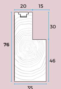
76mm L FRAME F/F 4008C
