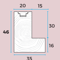
46mm L FRAME F/F 4008A
